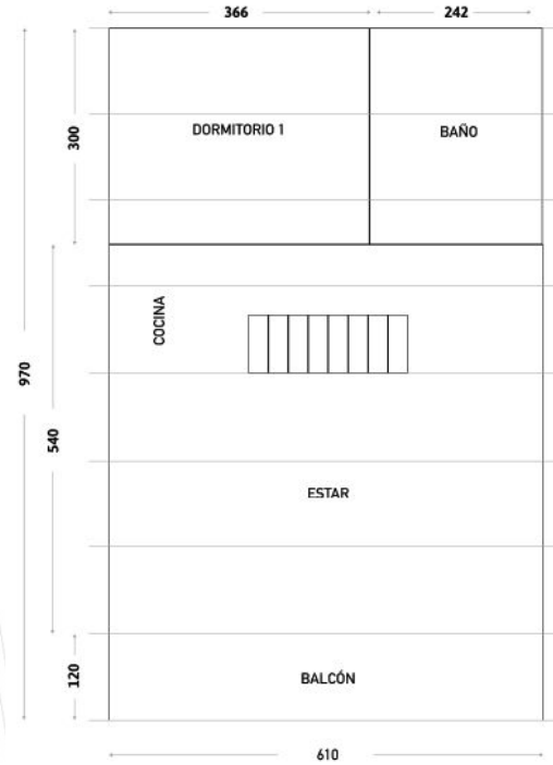
Piso 1
